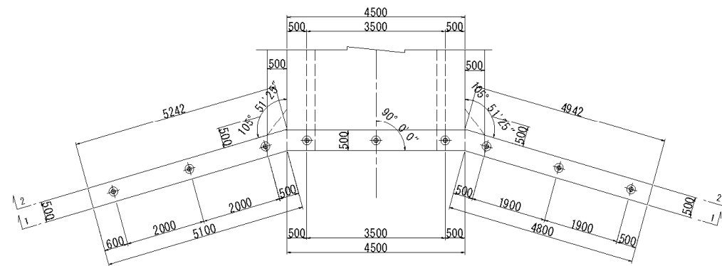
3 - 3
