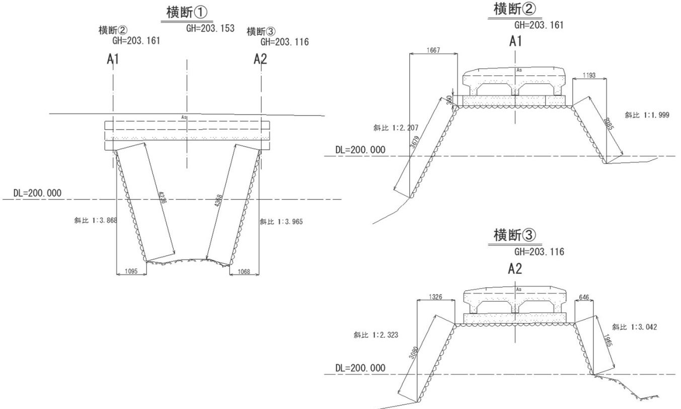
斜比算出根拠断面図
