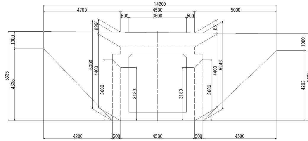
6 - 6
