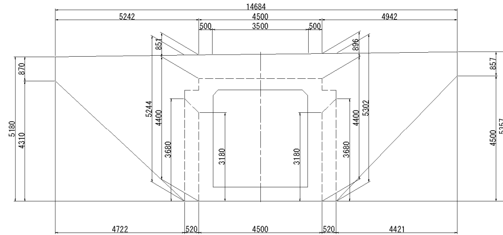
3 - 3
