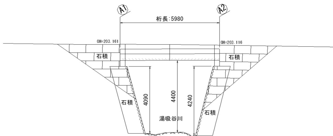
側 面 図
